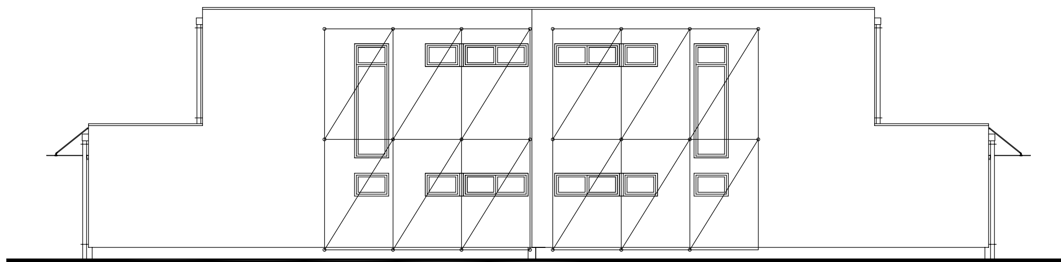
Pohled severní
